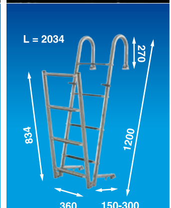
Rör /Tube \phi 32 mm
