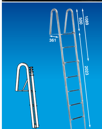
Rör /Tube \phi 38 mm
